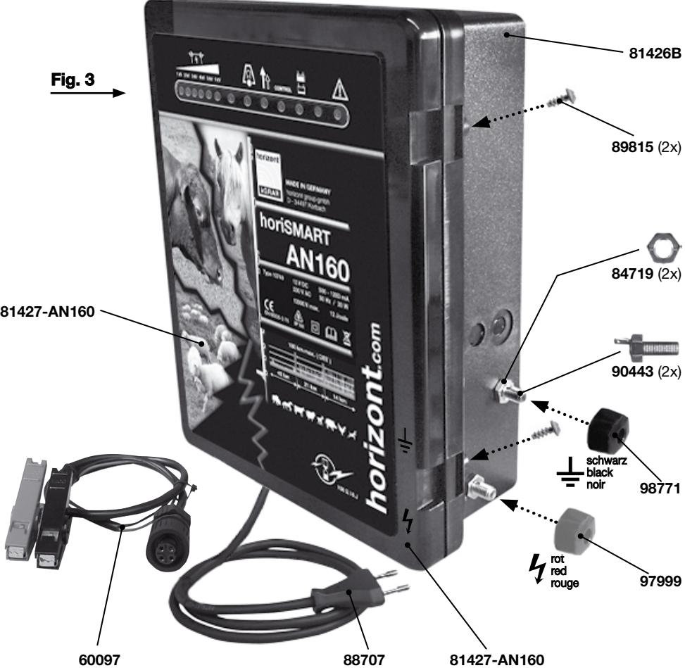
Fig. 2 Ersatzteile, Spare parts, Pièces détachées
