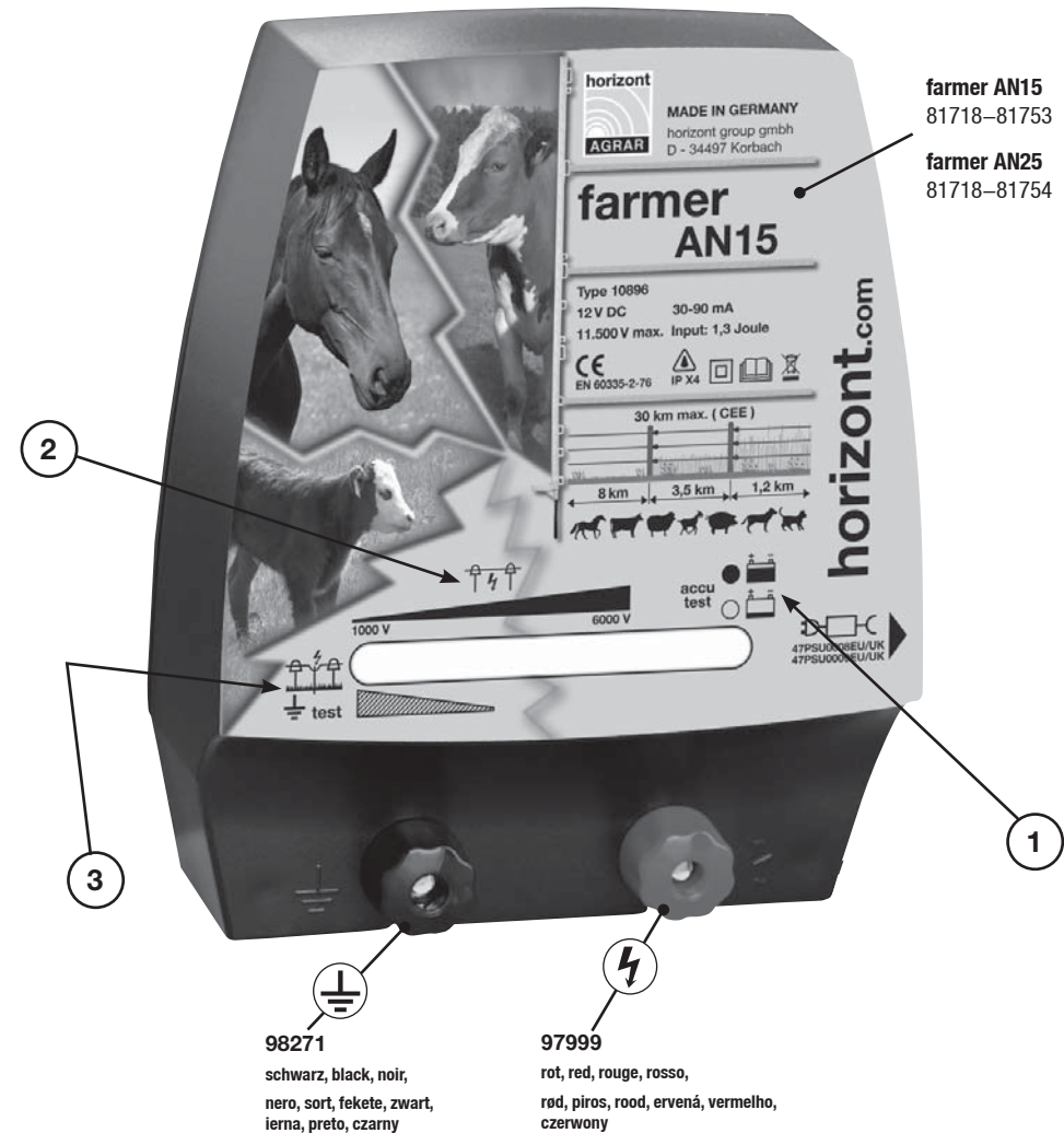
Fig. 2 Ersatzteile | Spare parts | Pièces détachées | Pezzi di ricambio Reservedele | Reserve onderdelen | Náhradné diely | Peças | Czci zapasowe
