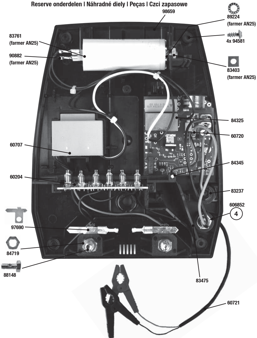
Fig. 1 Ersatzteile | Spare parts | Pièces détachées | Pezzi di ricambio Reservedele | Reserve onderdelen | Náhradné diely | Peças | Czci zapasowe
